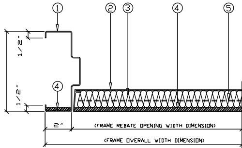
SECTION 'A'
