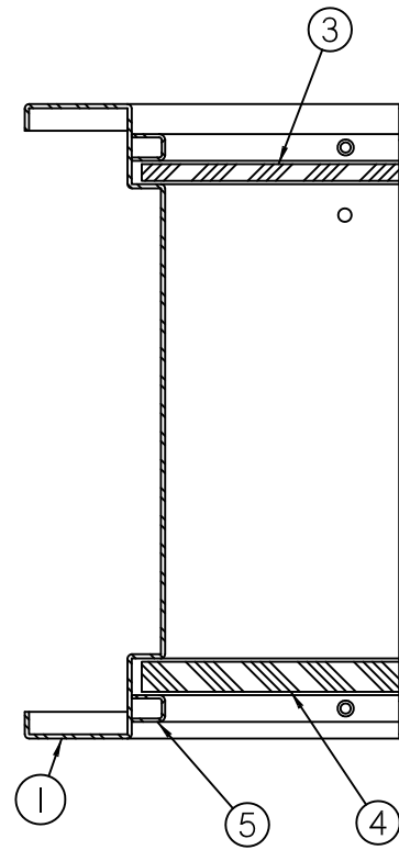
SECTION A-A
